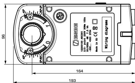
Привод
