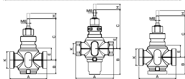
VLE122
