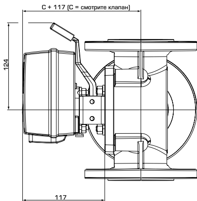
Установочные размеры для приводов серии CRC120 со смесительными клапанами ESBE серий MG, G, F, T/TM, H/HG и BV
