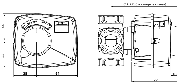
Установочные размеры для контроллеров серии CRA110 со смесительными клапанами ESBE VRG100, VRG200, VRG300, VRH100 и VRB100
