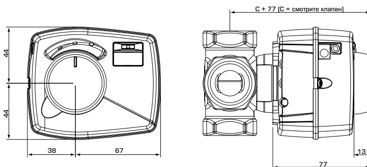
Установочные размеры для контроллеров серии CRC110 со смесительными клапанами ESBE VRG100, VRG200, VRG300, VRH100 и VRB100
