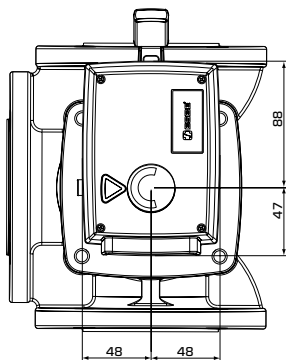
Установочные размеры для приводов серии CRC120 со смесительными клапанами ESBE серий MG, G, F, T/TM, H/HG и BV
