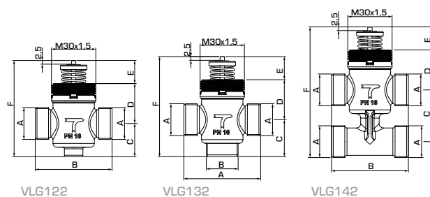
VLG122
